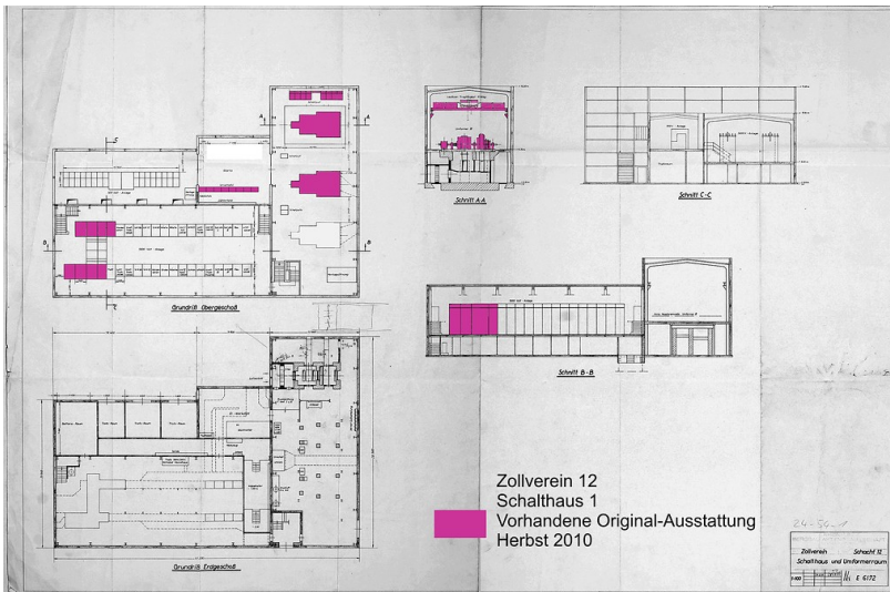
Plan der vorhandenen Original-Ausstattung des Schaltheim 1, Zollverein 12
