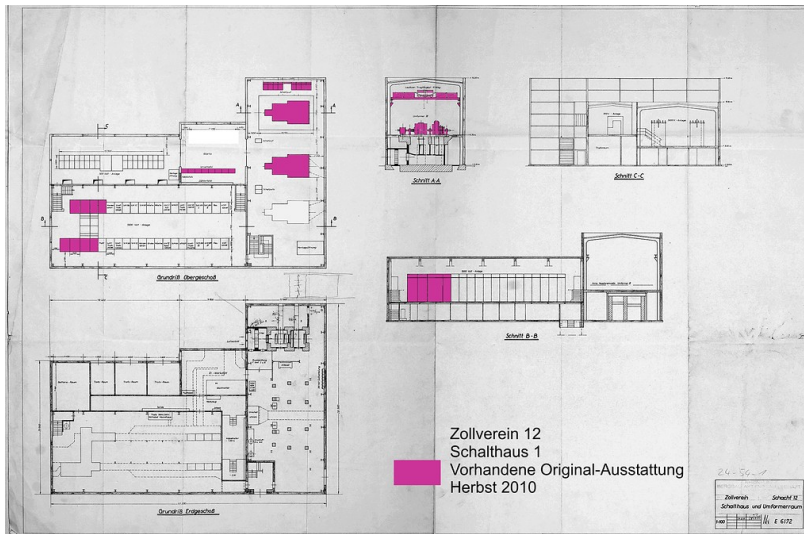
Plan der vorhandenen Original-Ausstattung des Schaltheus 1, Zollverein 12
