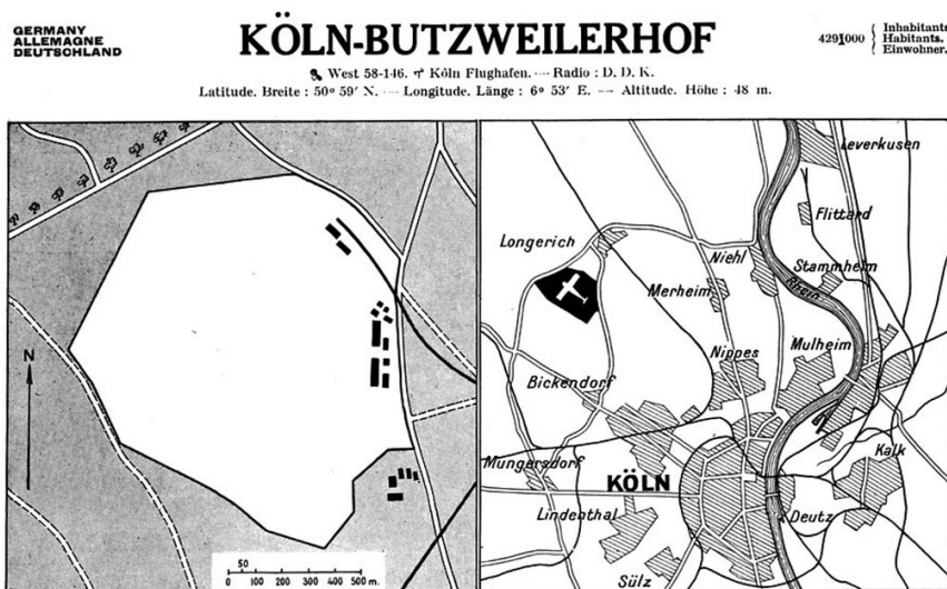
Lageplan und Kurzbeschreibung des Flugplatzes Köln-Butzweilerhof im Internationalen Flughandbuch von 1931, "International Air Guide: The reference book on civil and commercial aviation (Air atlas)" Fotograf/Urheber: unbekannt
