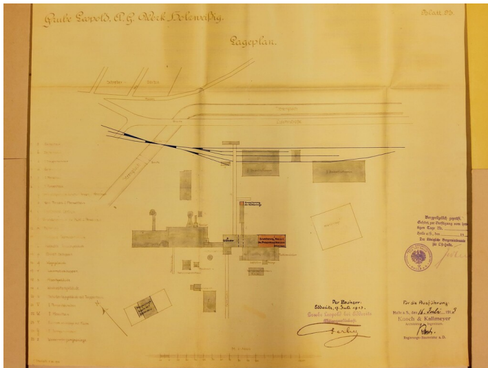
Altstandort Brikettfabrik Holzweißig - Lageplan Brikettfabrik Grube Leopold AG Werk Holzweißig von 1913 ( Kreismuseum Bitterfeld Sig. VIII C 1594) Fotograf/Urheber: NAME FEHLT
