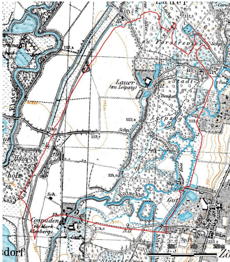
Tagebau Cospuden, Messtischblatt 1940 (Kartengrundlage: GeoSN, dl-de/by-2-0.: Historische Karten (Messtischblatt vor 1945).) Fotograf/Urheber: Ullrich Ochs
