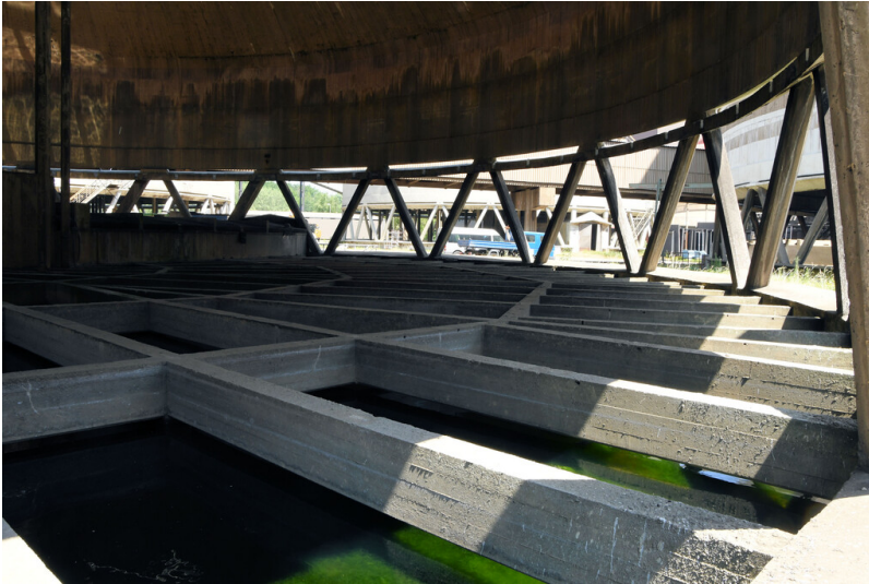
Kraftwerk Weisweiler: Kühlturm 6, Asbestzementeinbauten; Foto: 13.06.2023 Fotograf/Urheber: Dr. Norbert Gilson
