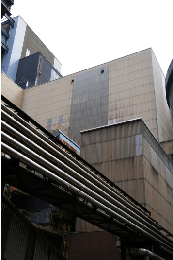
Kraftwerk Niederaußem: Kesselhaus Block F, Ansicht von Nordwesten; Foto: 15.08.2023 Fotograf/Urheber: Dr. Norbert Gilson
