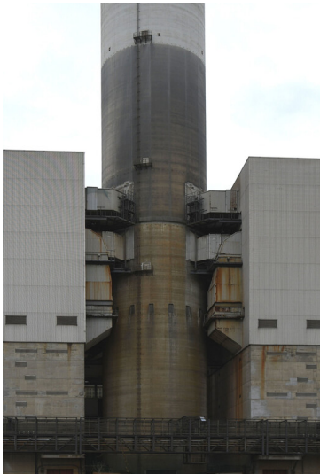
Kraftwerk Frimmersdorf II: Reingaseinleitungen in REA-Kamin 2, Ansicht von Westen; Foto: 22.03.2023 Fotograf/Urheber: Dr. Norbert Gilson
