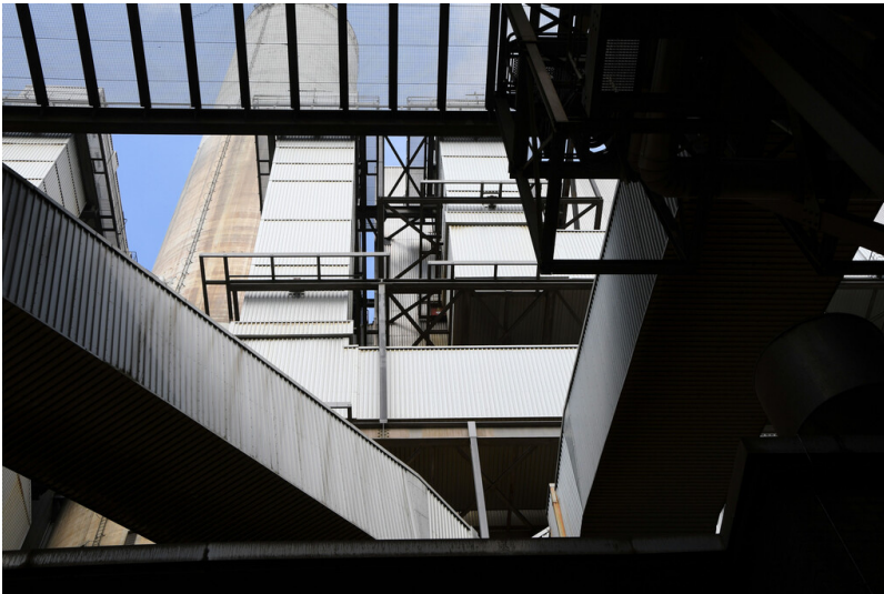
Kraftwerk Frimmersdorf II: Rohgaskanäle Blöcke E und F vor Kamin 1 und Wäschergebäude E/F/G/H, Ansicht von Osten; Foto: 23.06.2023 Fotograf/Urheber: Dr. Norbert Gilson
